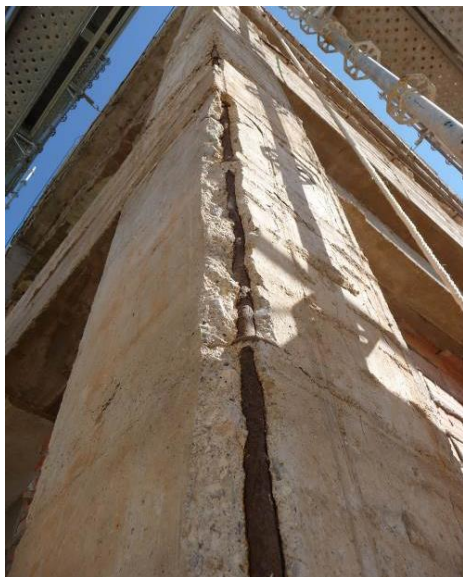
Fig. 8 y 9. Desprendimiento del hormigón por corrosión de armaduras en soportes
