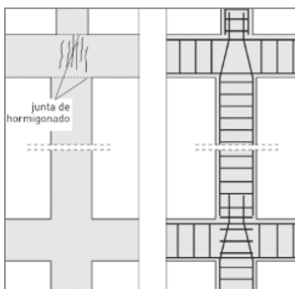
Fig. 15. Fisuración vertical en nudos de pórticos.
