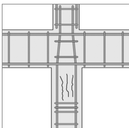
Fig. 17. Fisuración vertical en cabeza de pilar
