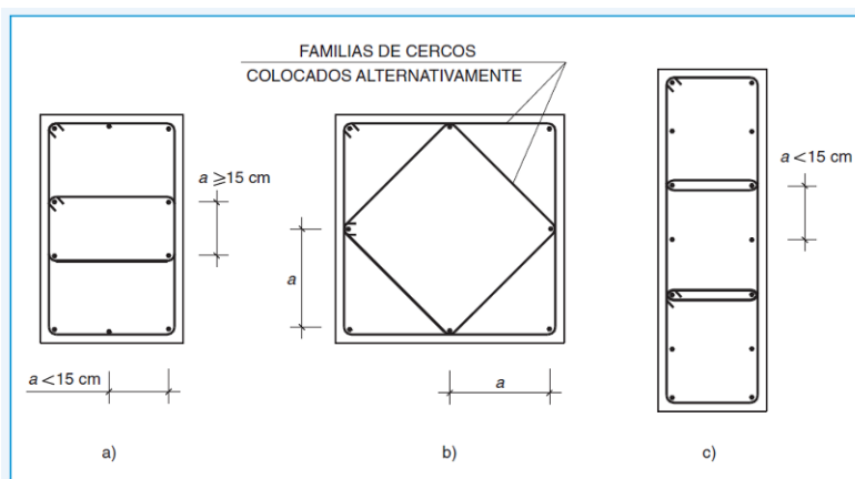
Fig. 20. Colocación de cercos en soportes
