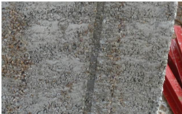
Fig. 5. Nidos de grava en soportes
