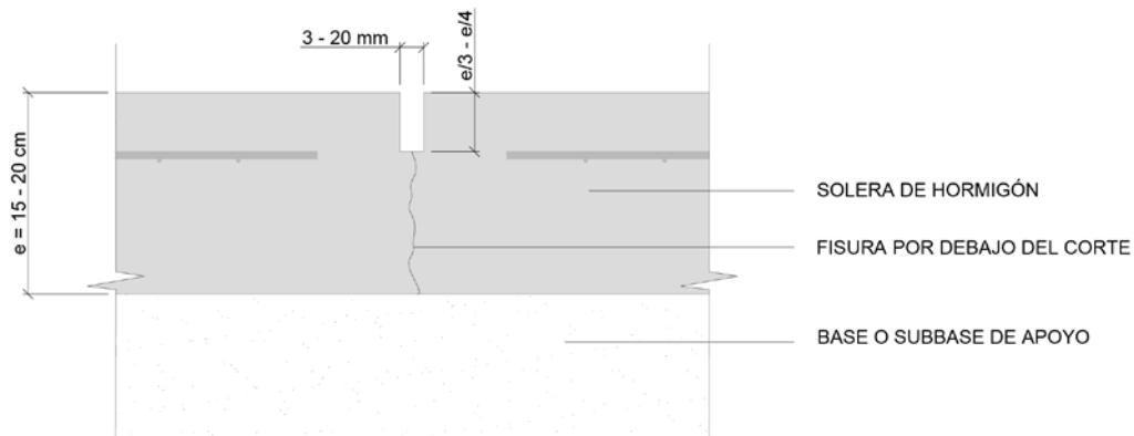
Fig. 9. Detalle junta de retracción por serrado
