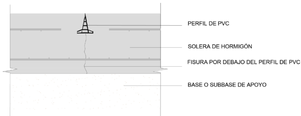
Fig. 10. Detalle junta de retracción con perfil de PVC
