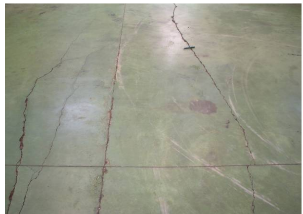
Fig. 6. Pérdida de apoyo localizado en la base
