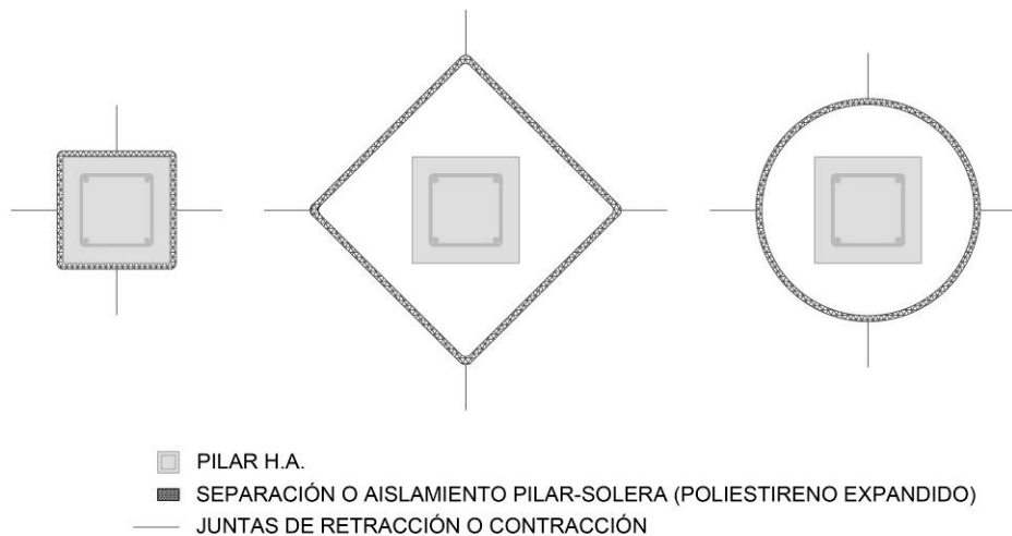
Fig. 8. Detalle juntas de separación o aislamiento entre la solera y otros elementos constructivos
