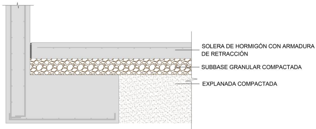
Fig. 7. Detalle encuentro solera con elementos de cimentación
