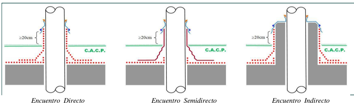
Fig. 6: Esquemas de los diferentes formatos de encuentros con elementos pasantes
