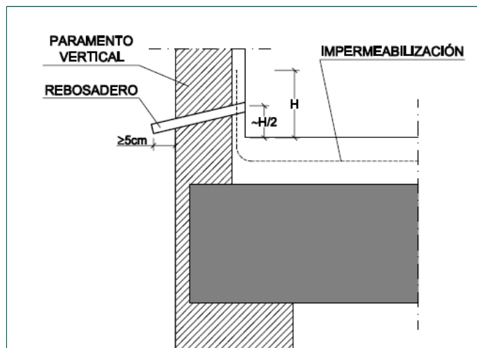
Fig. 3: Esquema de disposición de un rebosadero
