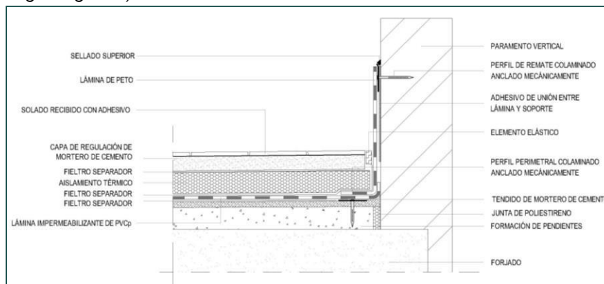
Fig. 5: Solución para encuentro de lámina de PVC-P con un paramento vertical
