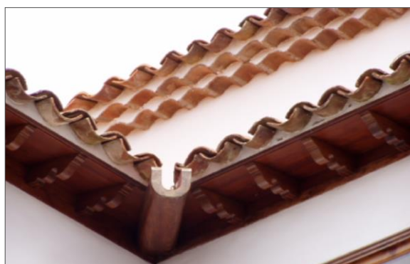
Fig. 2: Encuentro entre el frente de un alero y una limahoya
