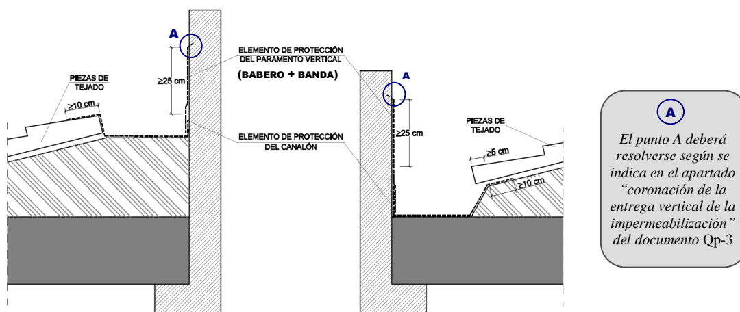
Fig. 9: Esquema del encuentro de un canalón empotrado con un faldón de cubierta inclinada:
