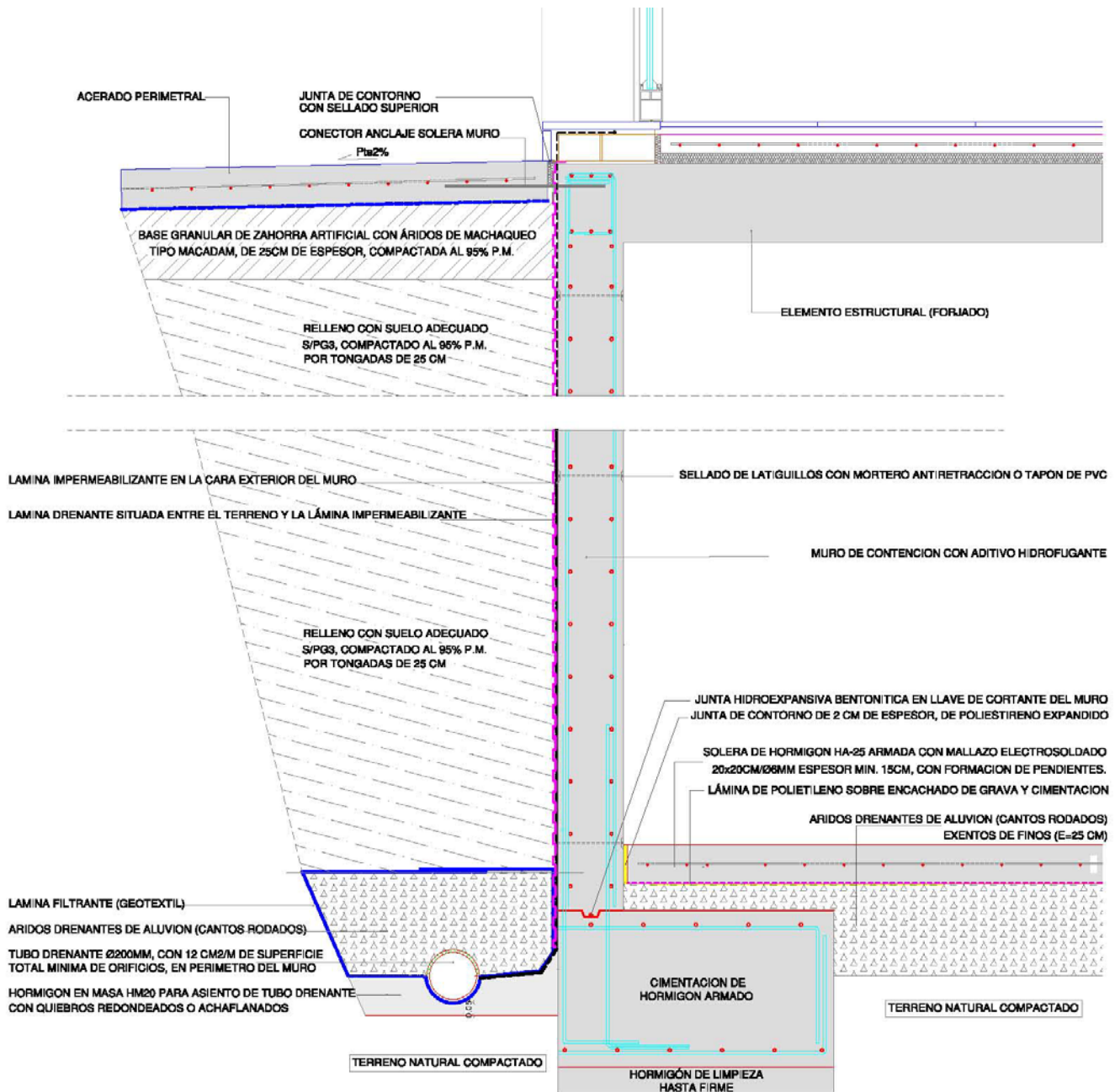
Fig. 7: Esquema orientativo sobre la impermeabilización, protección y drenaje de muro de sótano. Sin presencia de N.F.
