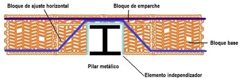
Fig. 11: Disposición de la fábrica de bloques cerámicos y del armado de refuerzo, en el encuentro con un pilar metálico
