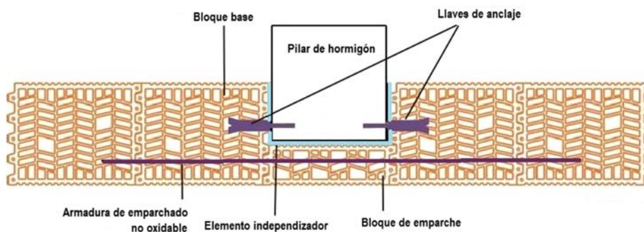
Fig. 12: Encuentro de una fábrica de bloques cerámicos aligerados con un pilar central de hormigón.
