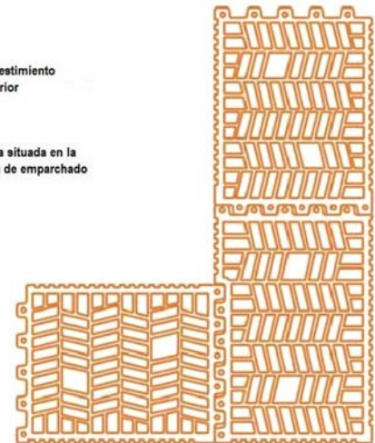
Fig. 10: Colocación de los bloques base en la esquina de un edificio, apreciándose el enjarje entre piezas.
