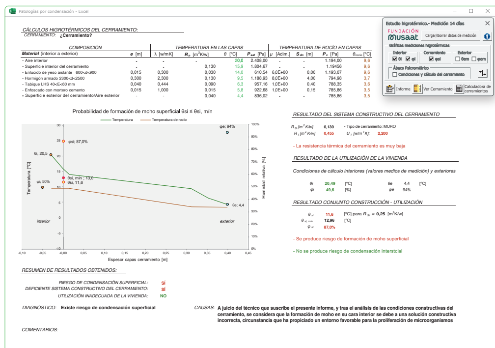
Imagen 71. Resultados del cálculo del cerramiento con los resultados medios de \theta_i y \phi_i .
