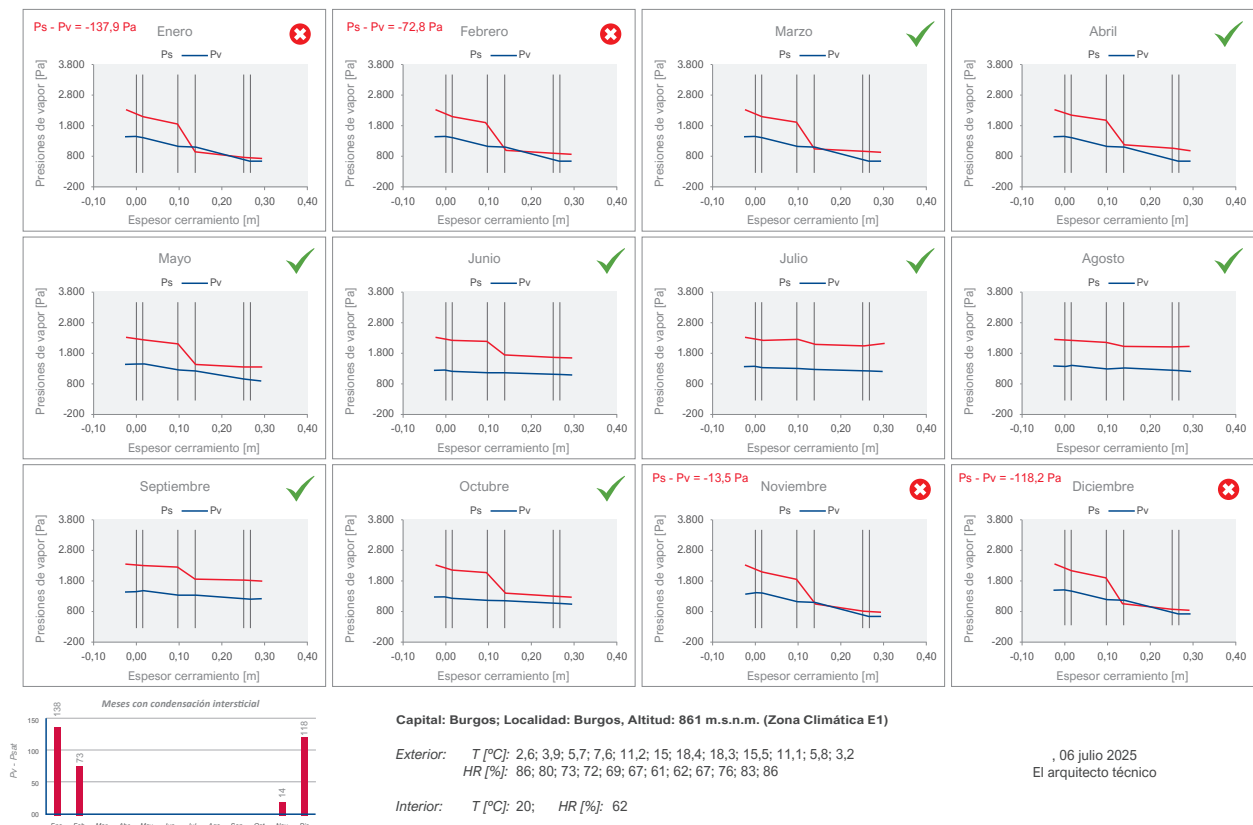
Imagen 128. Condensaciones intersticiales mes a mes.
