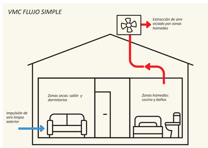
Imagen 107. VMC de flujo simple.
