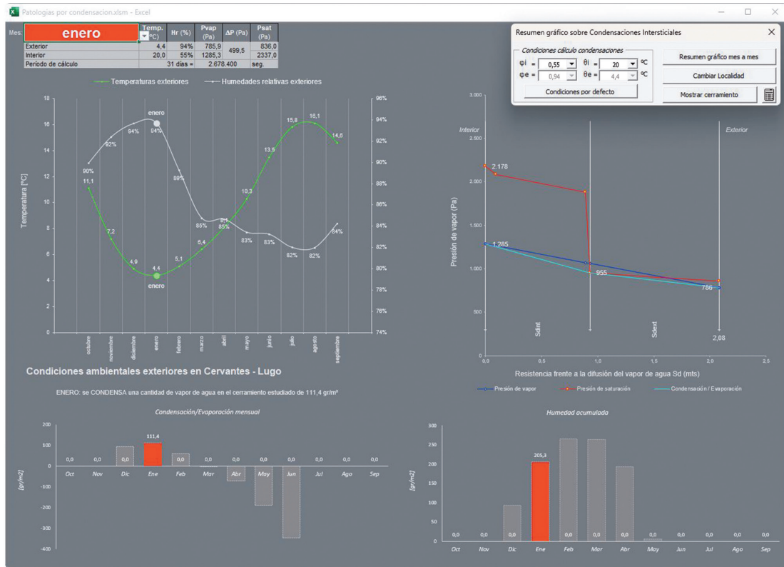
Imagen 139. Condensación/evaporación UNE EN ISO 13788:2001.
