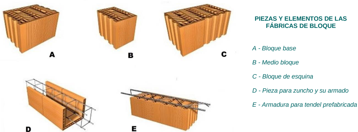
Fig. 5: Vista de algunos tipos y piezas especiales para las fábricas de bloque cerámico aligerado multialveolar
