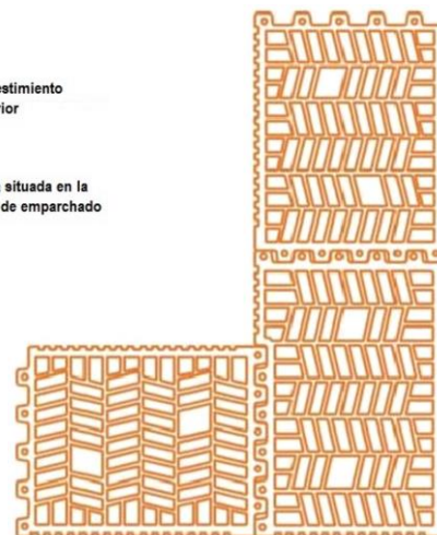
Fig. 10: Colocación de los bloques base en la esquina de un edificio, apreciándose el enjarje entre piezas.
