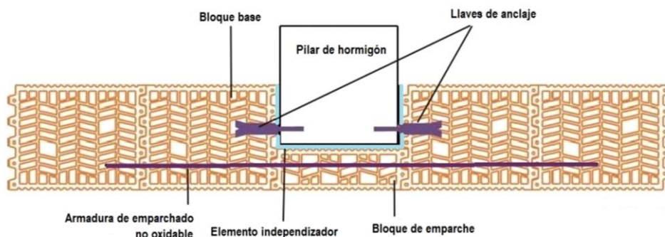
Fig. 12: Encuentro de una fábrica de bloques cerámicos aligerados con un pilar central de hormigón.
