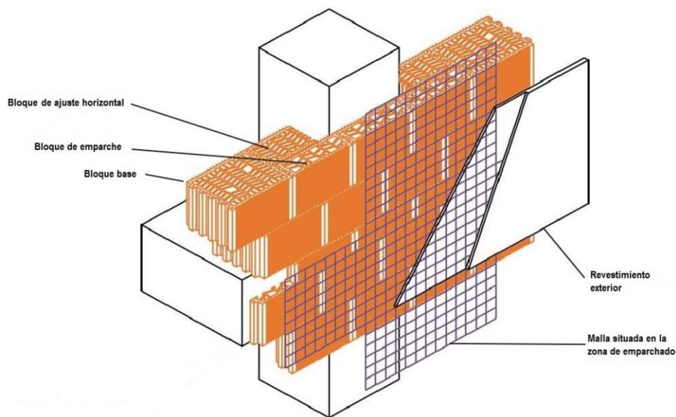
Fig. 8: Vista tridimensional de la primera hoja de bloques cerámicos con el borde de un pilar y el canto de un forjado.
