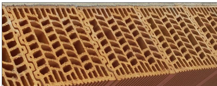
Fig. 6: Vista del machihembrado lateral de los bloques. Según este sistema, las piezas deben colocarse a tope y sin relleno de mortero de cemento en las juntas verticales.
