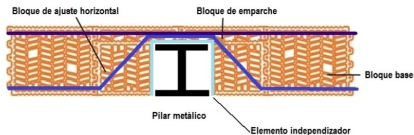
Fig. 11: Disposición de la fábrica de bloques cerámicos y del armado de refuerzo, en el encuentro con un pilar metálico
