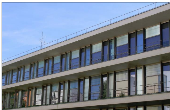
Fig.11: Fachada-panel con subestructura de aluminio anodizado y lunas de vidrio con áreas tintadas y no tintadas. Sobresale un voladizo con inclusión de vegetación sobre él
