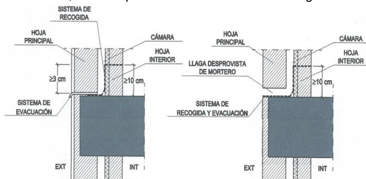
Fig. 3: Formas de resolución de la cámara de aire ventilada interior con el forjado
