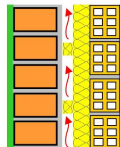
Fig. 4: Consecución constructiva de la CAVIC (cámara de aire ventilada interior de cerramiento), situada por delante de la capa aislante utilizando tacos de este mismo material
