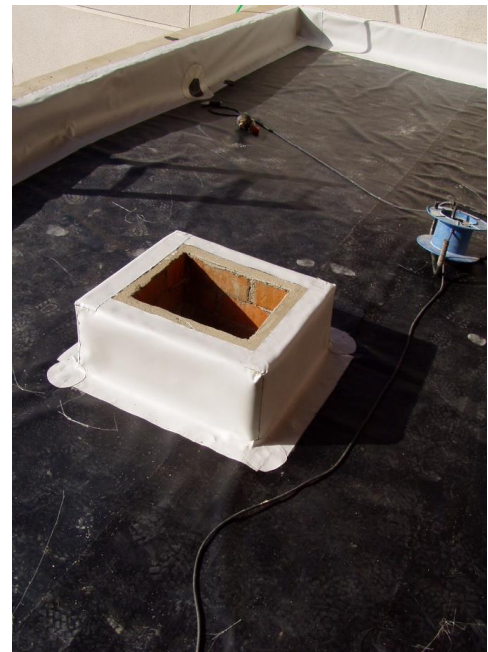
Fig. 4: Disposición de una lámina impermeabilizante de PVCp (la de color blanco, es resistente a la intemperie).
