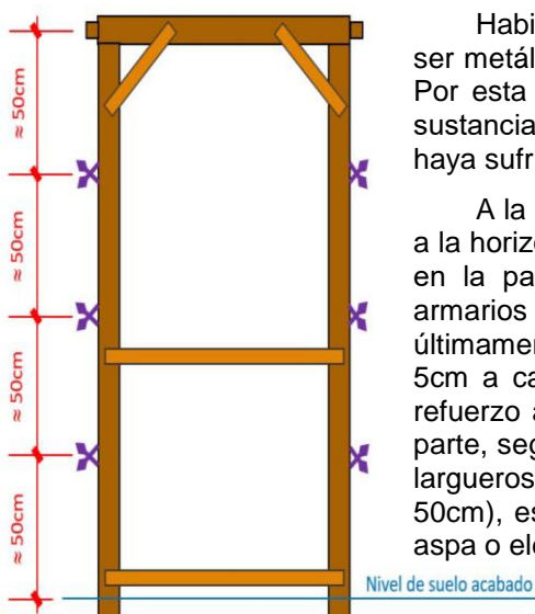
Fig. 4: Esquema de la configuración de un precerco de puerta, con indicación de las distancias entre patillas de anclaje.
