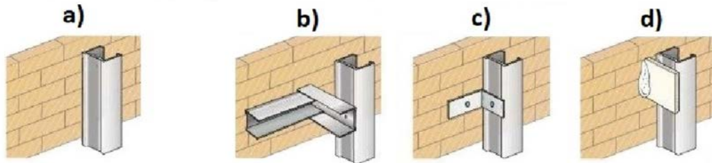
Fig. 5: Interrelación entre los montantes del trasdosado y el trasdós del muro-base. ▪ Montantes libres -no arriostrados- (a) ▪ Montantes arriostrados: con doblado de trozo de otro montante (b); con perfil angular (c); con lambeta o cartela (d).
