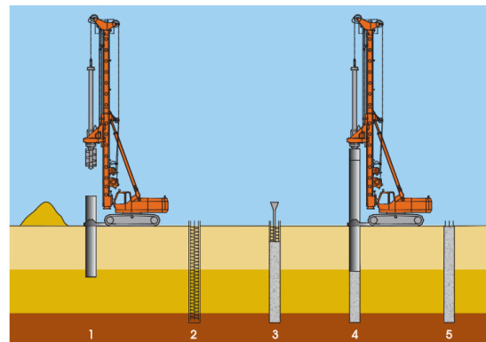
Figura 3: Pilote de extracción con entubación recuperable
