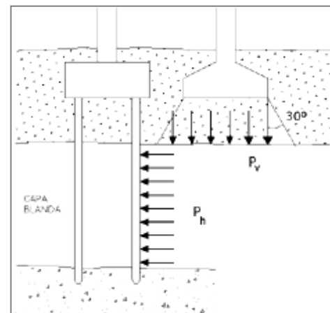
Figura 6: Empujes horizontales producidos por cargas superficiales
