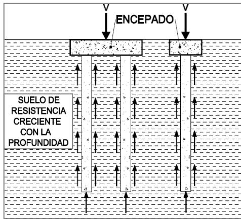
Figura 4. Pilotes por fuste
