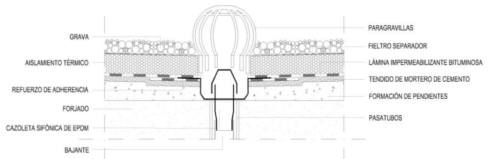
Fig. 5: Solución constructiva para un encuentro de cazoleta de EPDM con una lámina bituminosa (cubierta invertida no transitable)
