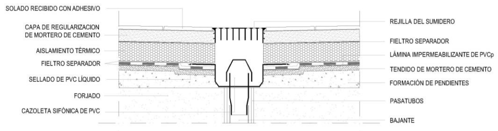
Fig. 6: Solución constructiva para un encuentro de cazoleta de PVC de ala flexible con una lámina de PVC-P (cubierta invertida transitable)
