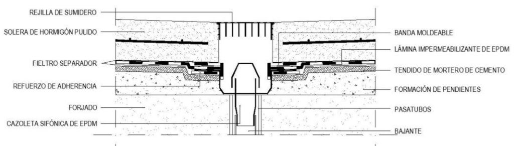
Fig. 7: Solución constructiva para un encuentro de cazoleta de EPDM con una lámina de igual material (cubierta transitable convencional no aislada)
