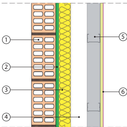
-Esquema 0- Vista en planta de las capas constituyentes de este tipo de fachada convencional de fábrica de ladrillo cara vista.
