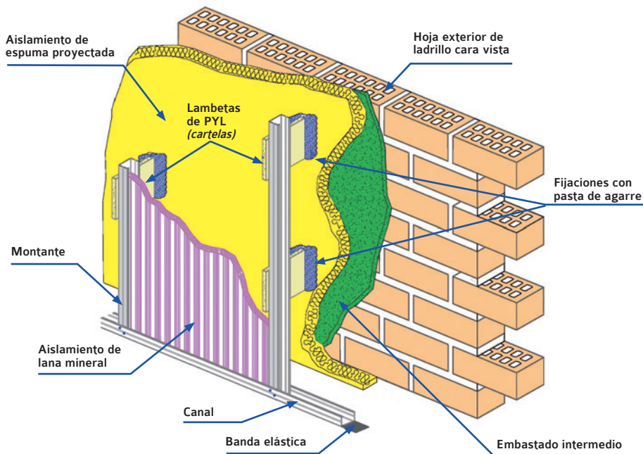
-Detalle 7- Realización del trasdosado autoportante de placas de yeso laminado. Arriostramiento con lambetas y colocación de una segunda capa de aislamiento entre montantes.
