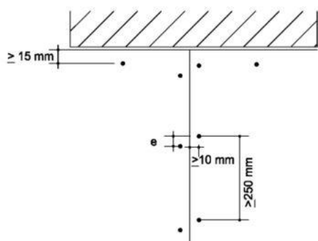
Fig. 10: Distancia entre tornillos placa-metal (25cm) y contrapeado de los tornillos a cada lado de la junta (e)
