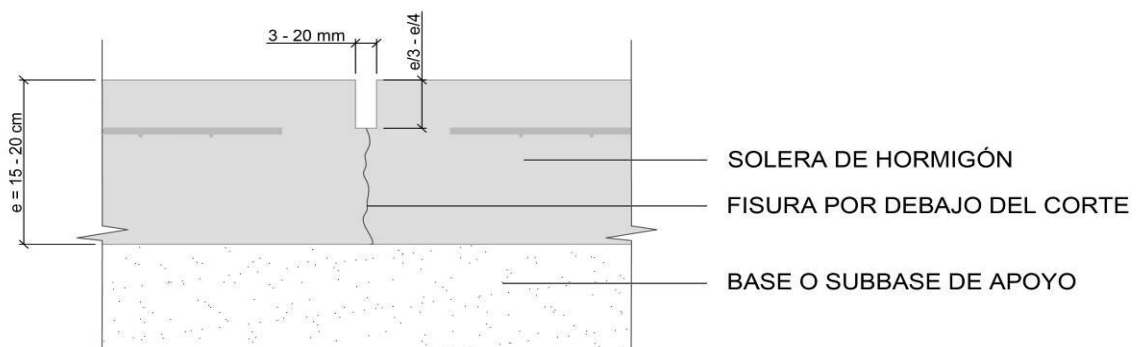
Fig. 13. Detalle junta de retracción por serrado
