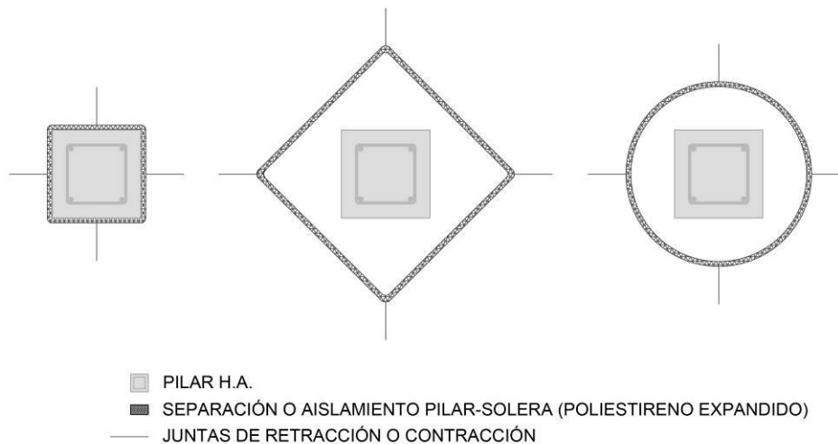
Fig. 12. Detalle juntas de separación o aislamiento entre la solera y otros elementos constructivos
