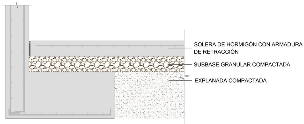
Fig. 11. Detalle encuentro solera con elementos de cimentación
