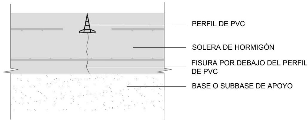
Fig. 14. Detalle junta de retracción con perfil de PVC
